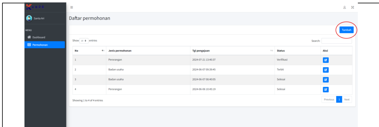
Gambar 4 Daftar permohonan
