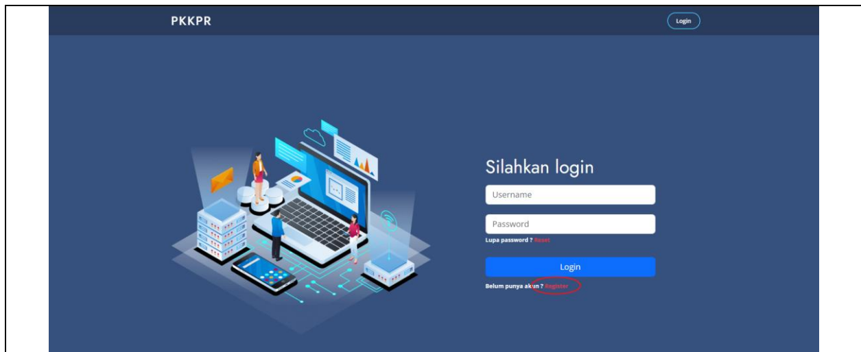
Gambar 1 Halaman login
